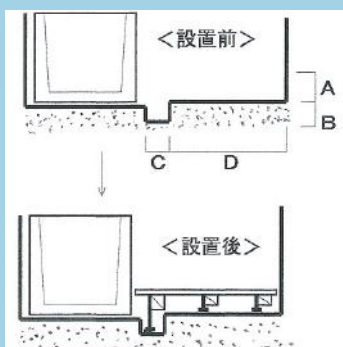
浴槽前に排水溝がある場合
