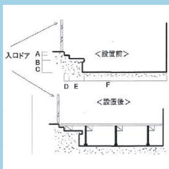
敷居部分 乗せ掛け型
